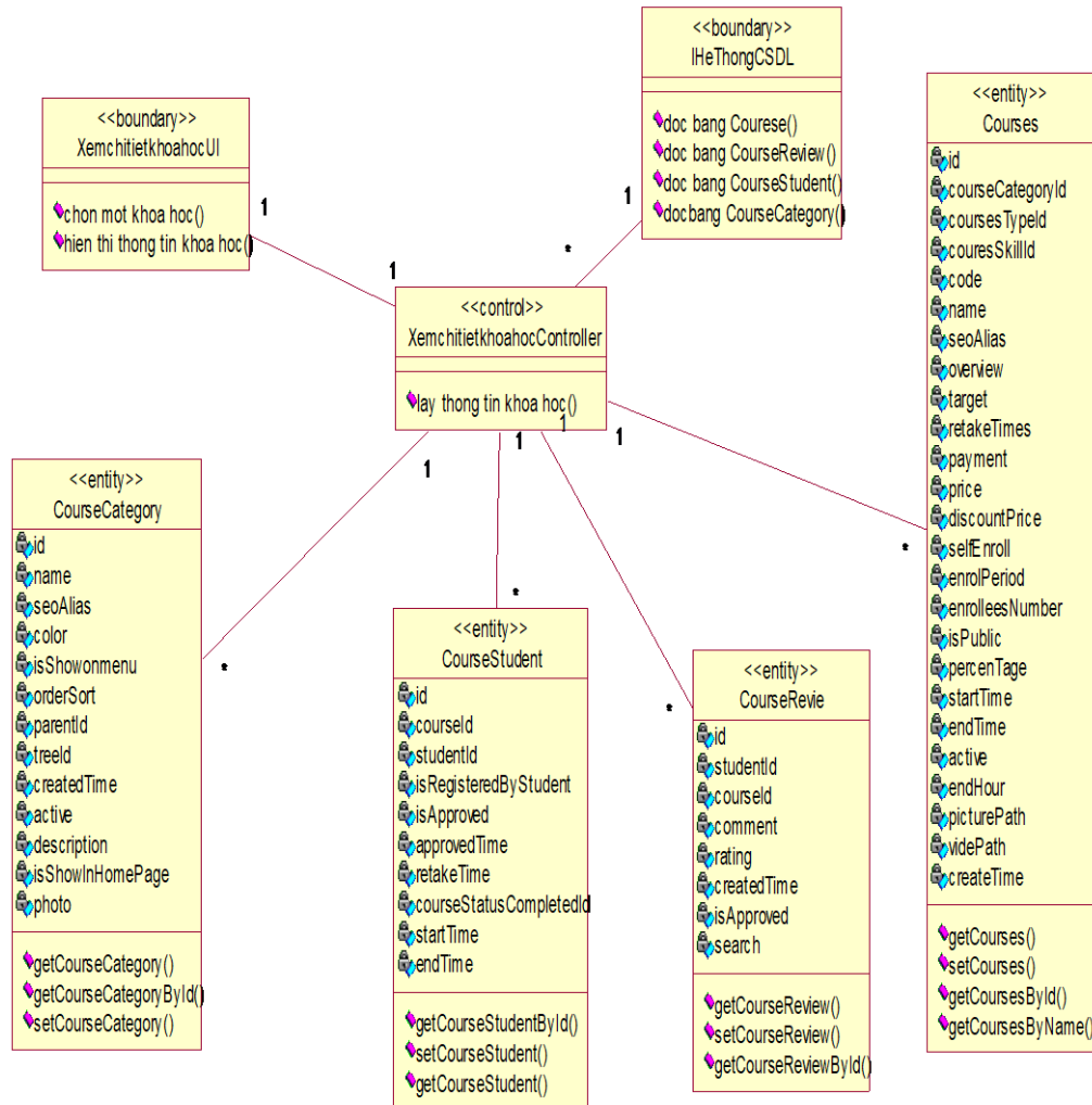
Hình 2.7. Biểu đồ lớp phân tích use case xem chi tiết khoá học
