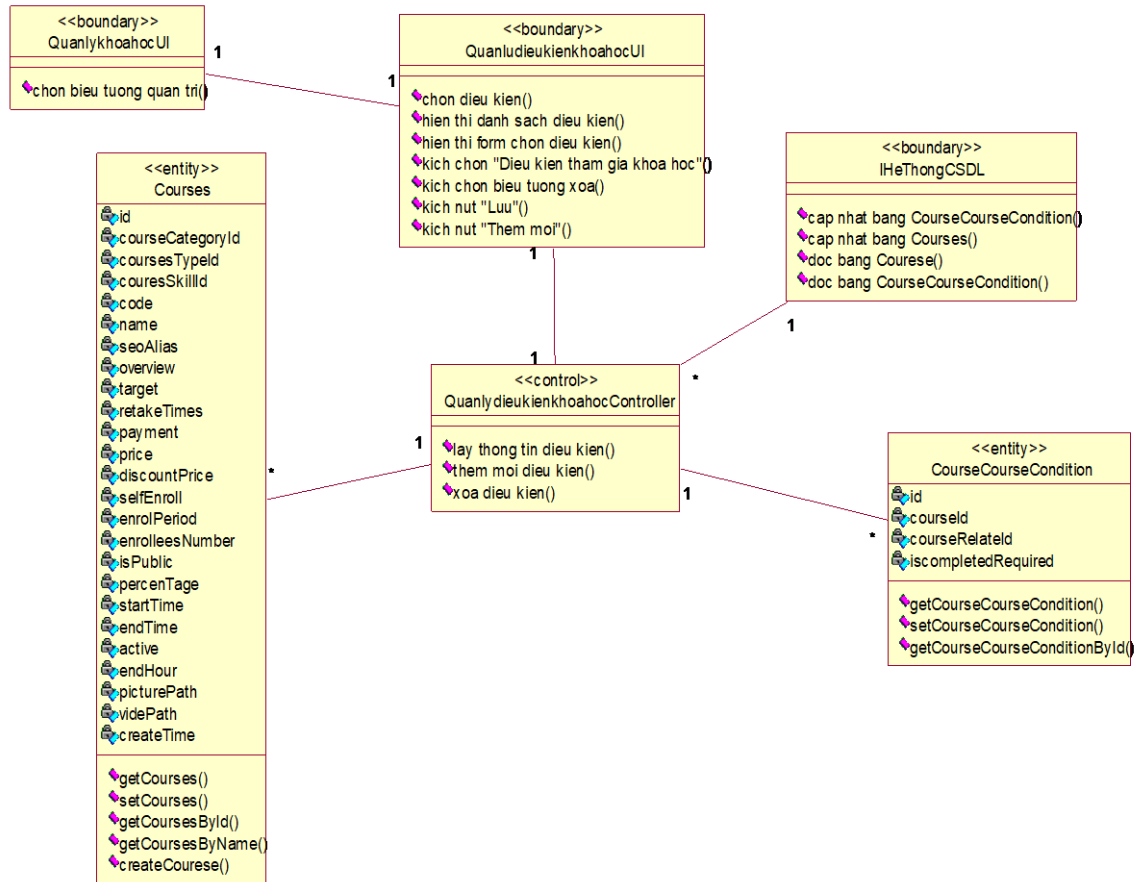
Hình 2.35. Biểu đồ lớp phân tích use case quản lý điều kiện tham gia khoá học trong chi tiết khoá học
