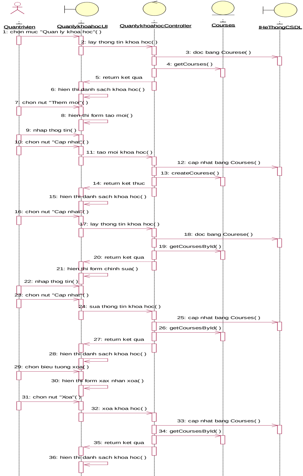
Hình 2.22. Biểu đồ trình tự use case quản lý khoá học
