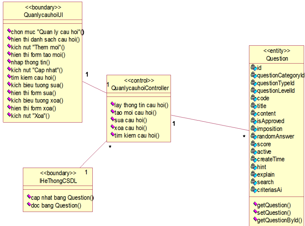
Hình 2.43. Biểu đồ lớp phân tích use case quản lý câu hỏi
