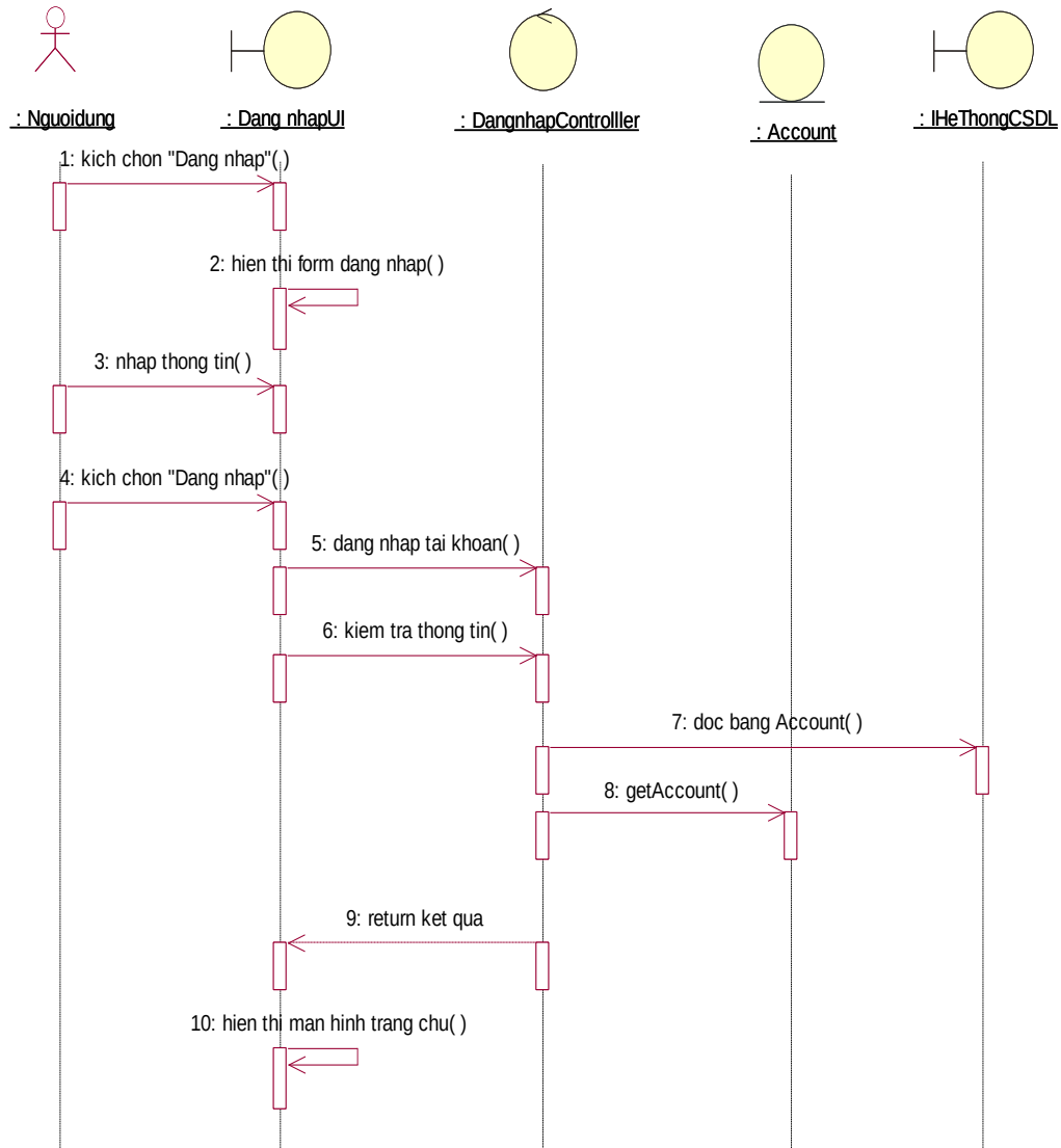
Hình 2.2. Biểu đồ trình tự use case đăng nhập
