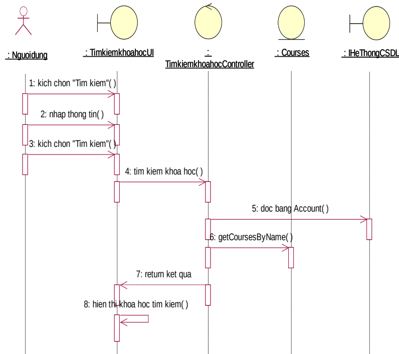
Hình 2.8. Biểu đồ trình tự use case tìm kiếm khoá học
