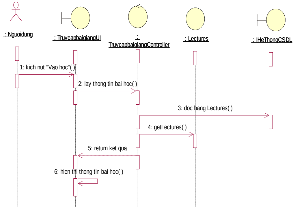
Hình 2.14. Biểu đồ trình tự use case truy cập bài giảng
