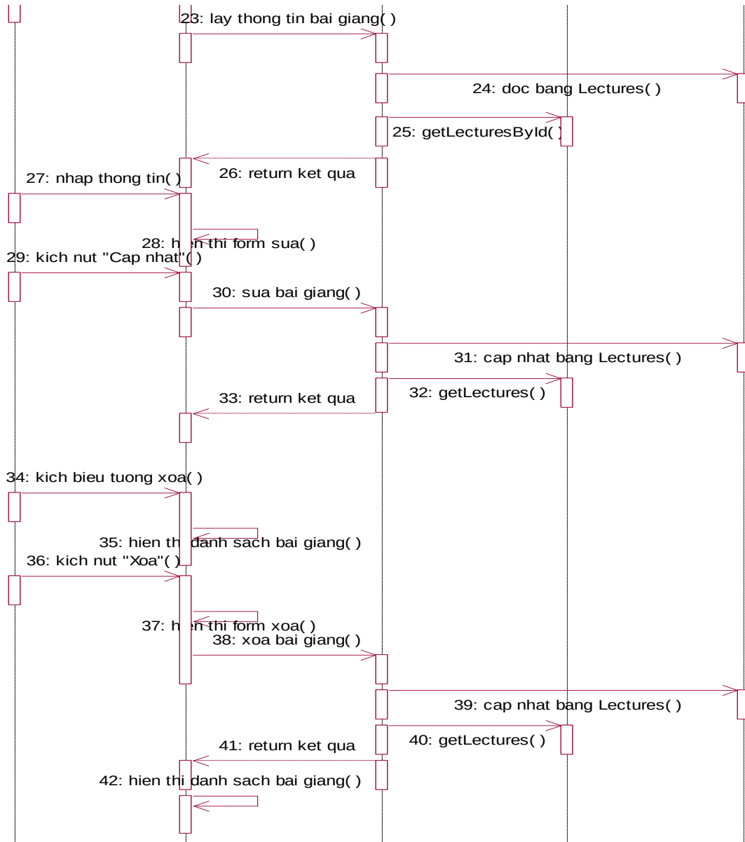
Hình 2.40. Biểu đồ trình tự use case xem quản lý bài giảng
