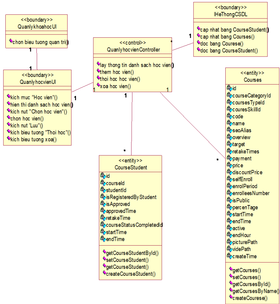
Hình 2.32. Biểu đồ lớp phân tích use case quản lý học viên trong chi tiết khoá học
