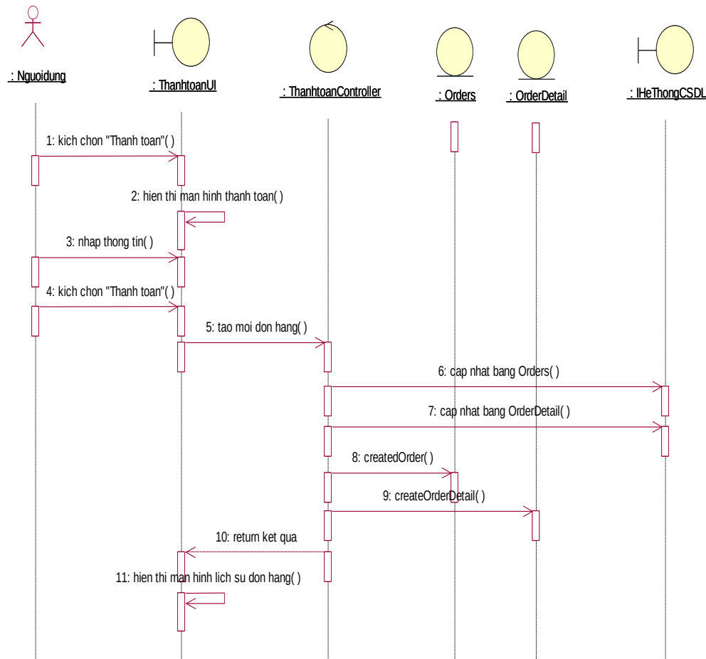
Hình 2.10. Biểu đồ trình tự use case thanh toán
