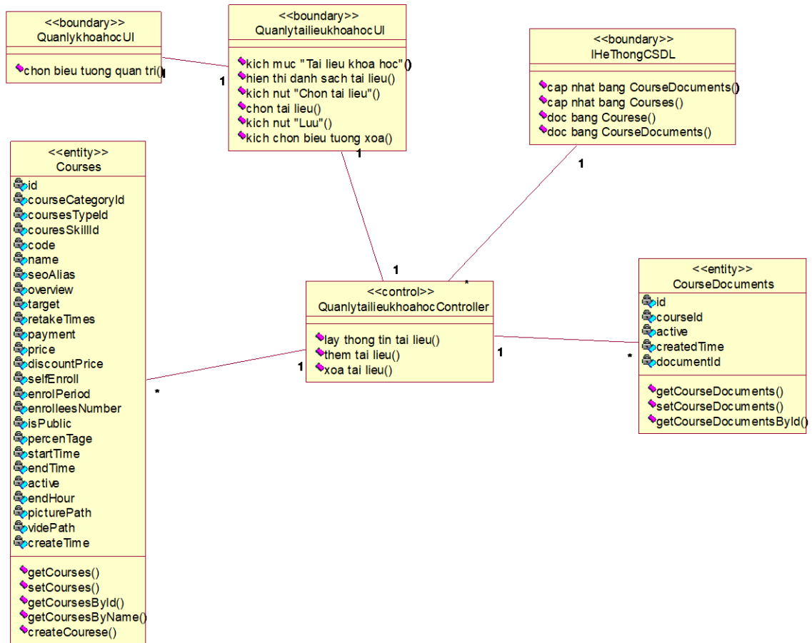
Hình 2.37. Biểu đồ lớp phân tích use case quản lý tài liệu trong chi tiết khoá học
