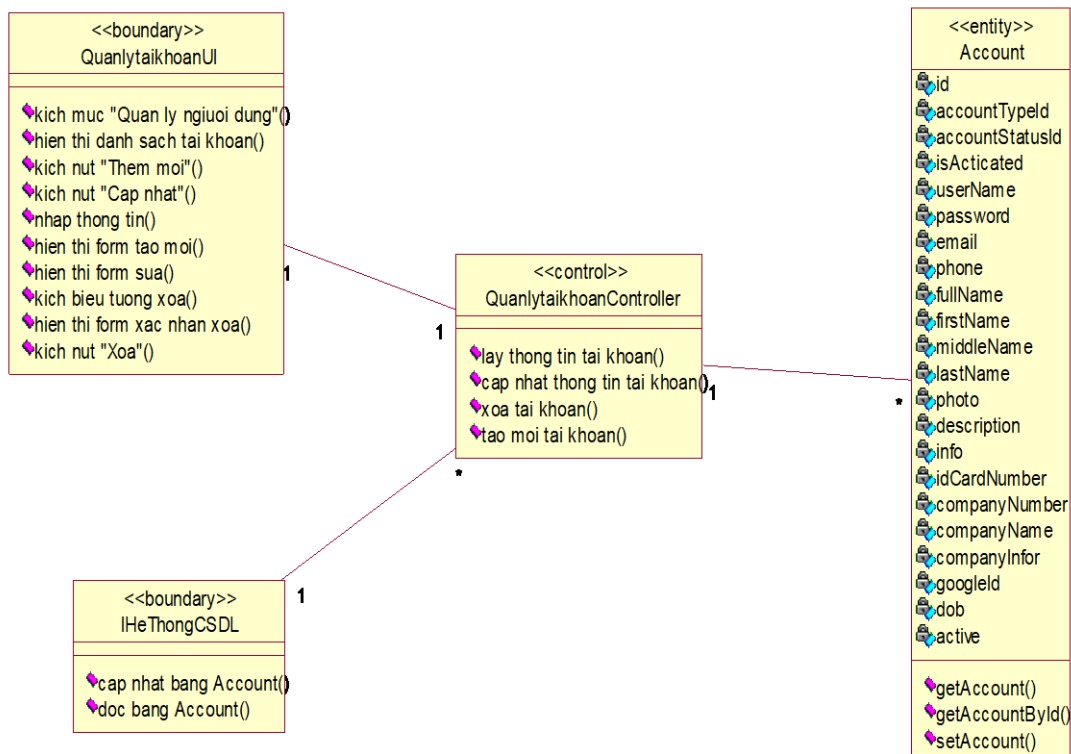
Hình 2.21. Biểu đồ lớp phân tích use case quản lý tài khoản/người dùng
