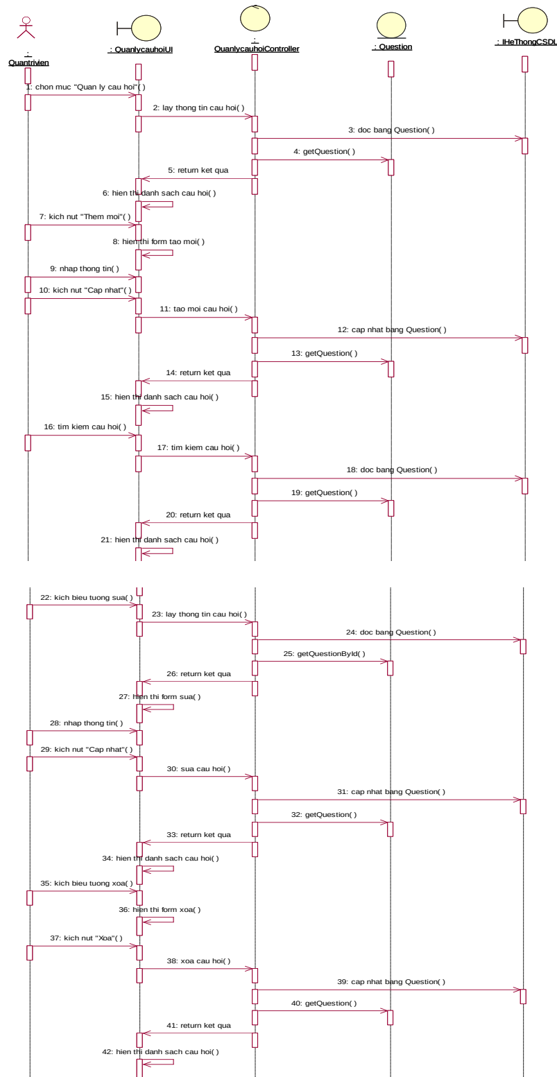
Hình 2.42. Biểu đồ trình tự use case quản lý câu hỏi
