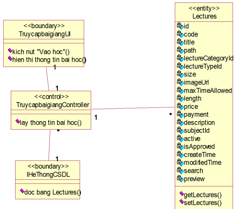
Hình 2.15. Biểu đồ lớp phân tích use case truy cập bài giảng
