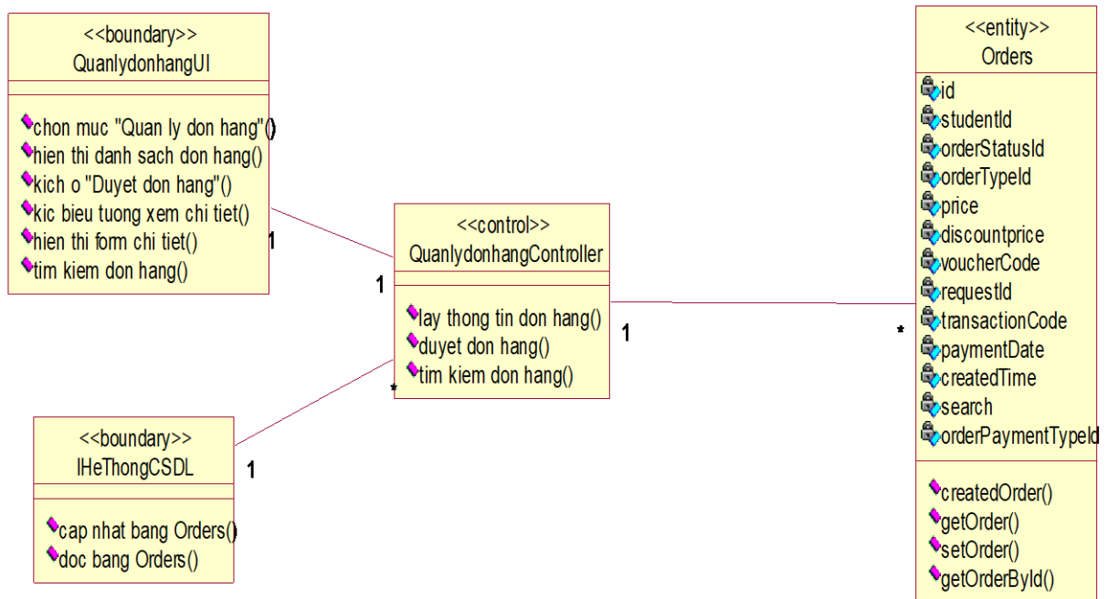
Hình 2.47. Biểu đồ lớp phân tích use case quản lý đơn hàng
