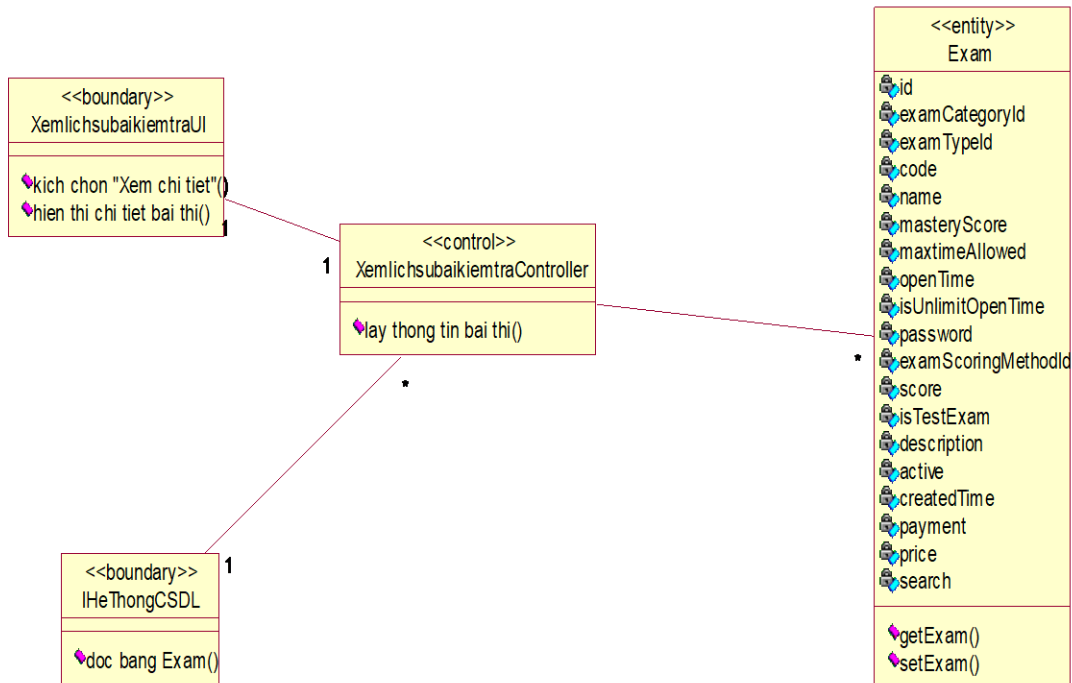
Hình 2.19. Biểu đồ lớp phân tích use case xem lịch sử bài kiểm tra/thi
