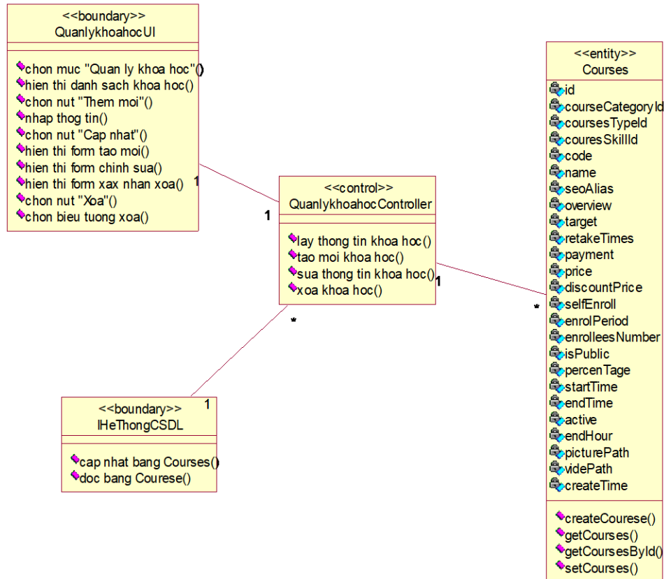
Hình 2.23. Biểu đồ lớp phân tích use case quản lý khoá học
