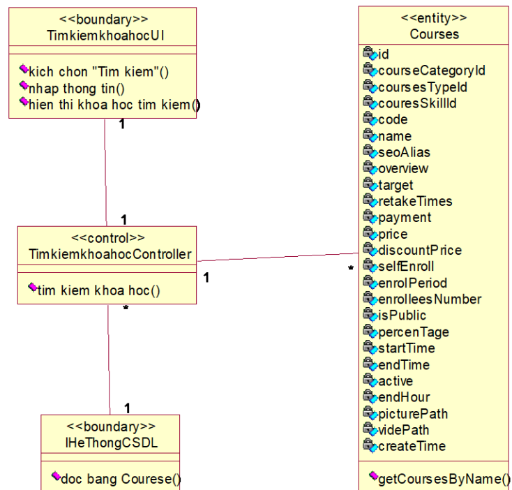
Hình 2.9. Biểu đồ lớp phân tích use case tìm kiếm khoá học
