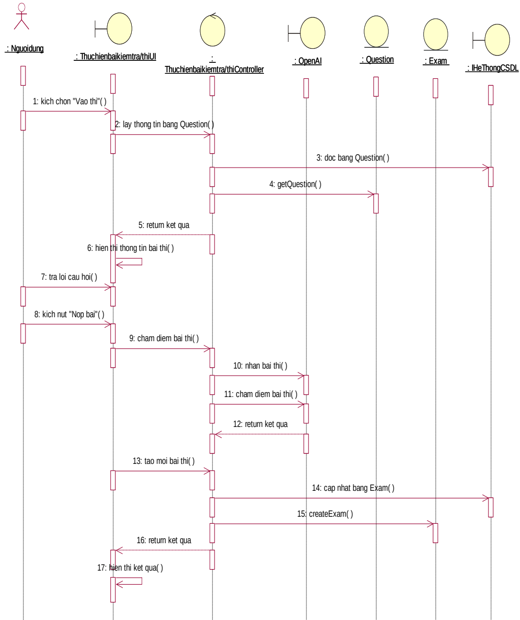
Hình 2.16. Biểu đồ trình tự use case thực hiện bài kiểm tra/thi
