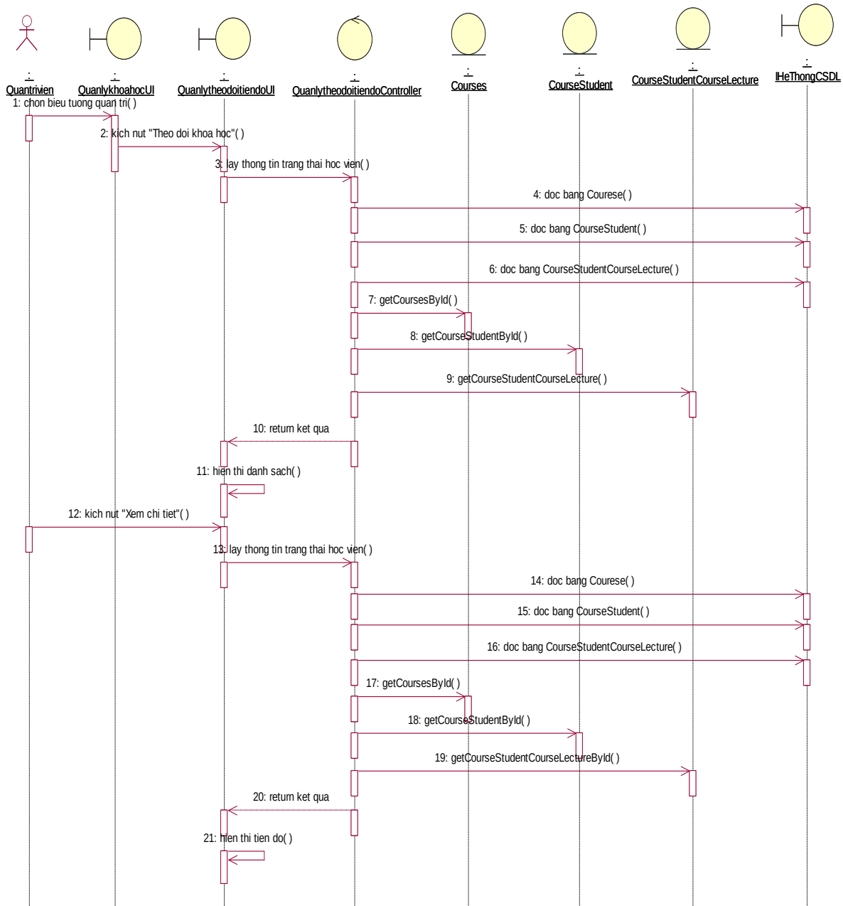
Hình 2.31. Biểu đồ trình tự use case theo dõi tiến độ học viên trong chi tiết khoá học
