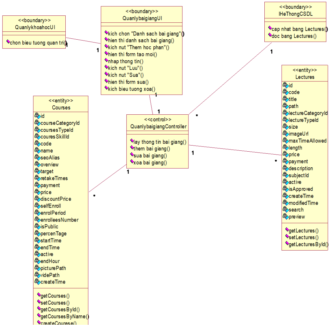
Hình 2.33. Biểu đồ lớp phân tích use case quản lý bài giảng trong chi tiết khoá học
