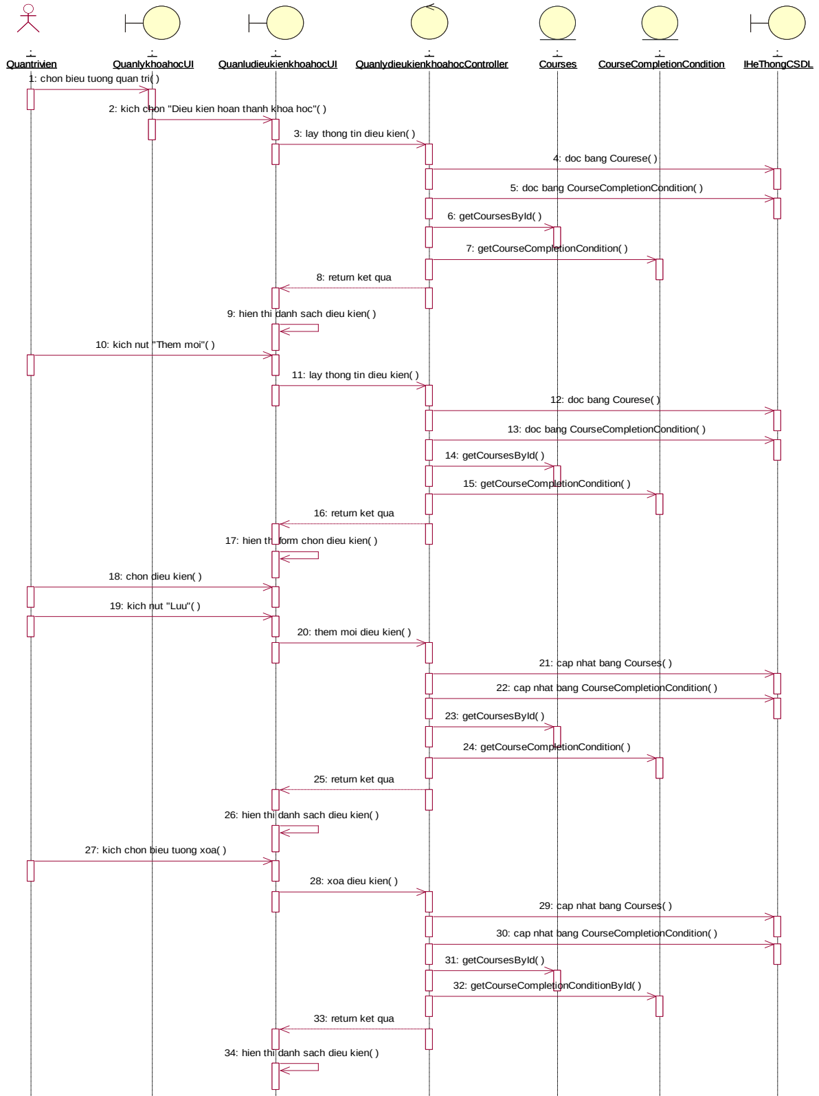
Hình 2.28. Biểu đồ trình tự use case quản lý điều kiện hoàn thành khoá học trong chi tiết khoá học
