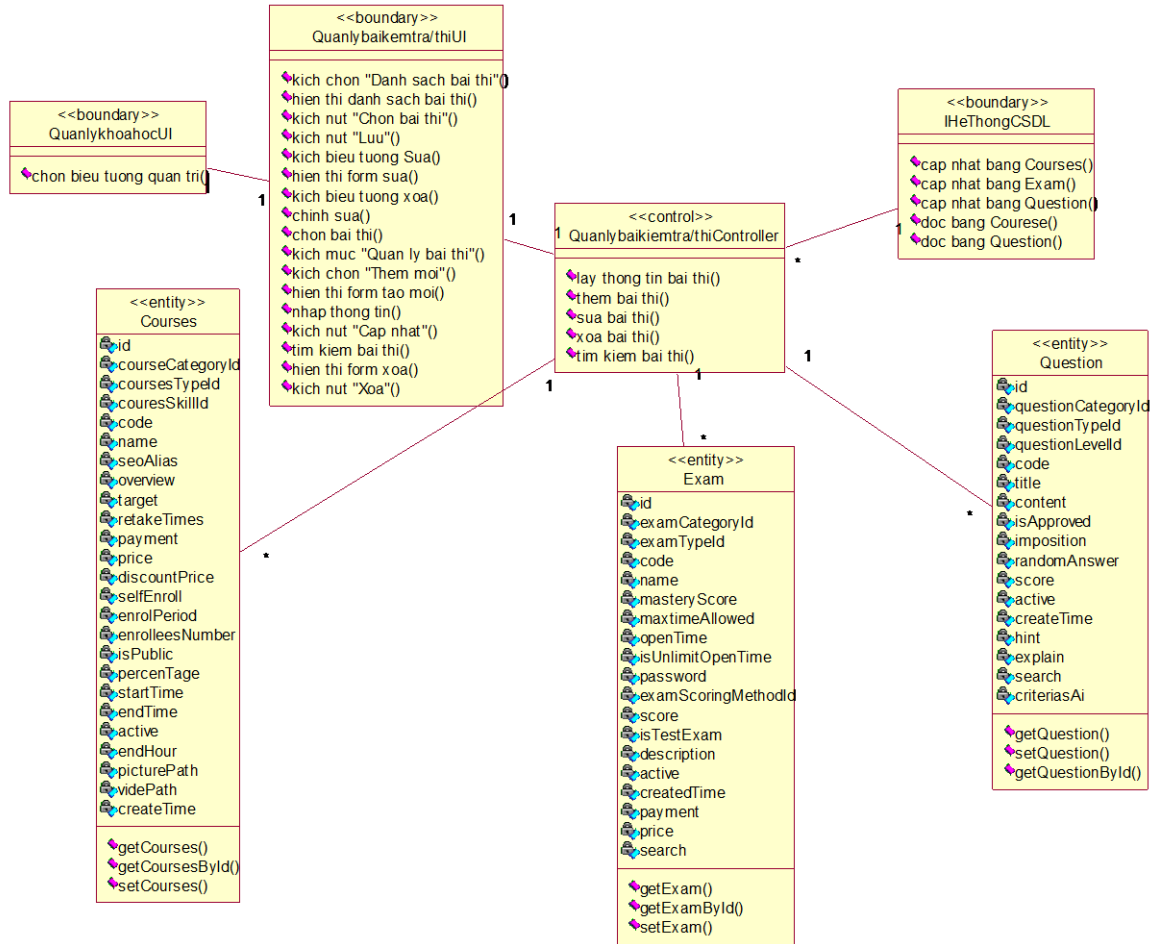
Hình 2.34. Biểu đồ lớp phân tích use case quản lý bài kiểm tra/thi trong chi tiết khoá học
