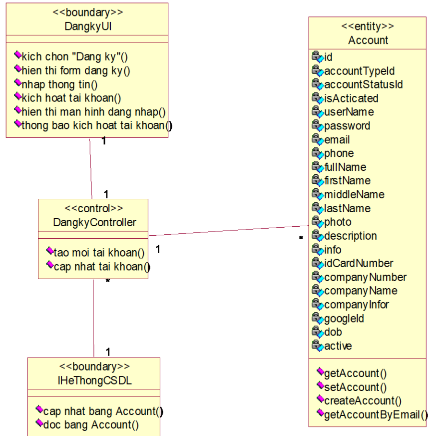
Hình 2.5. Biểu đồ lớp phân tích use case đăng ký
