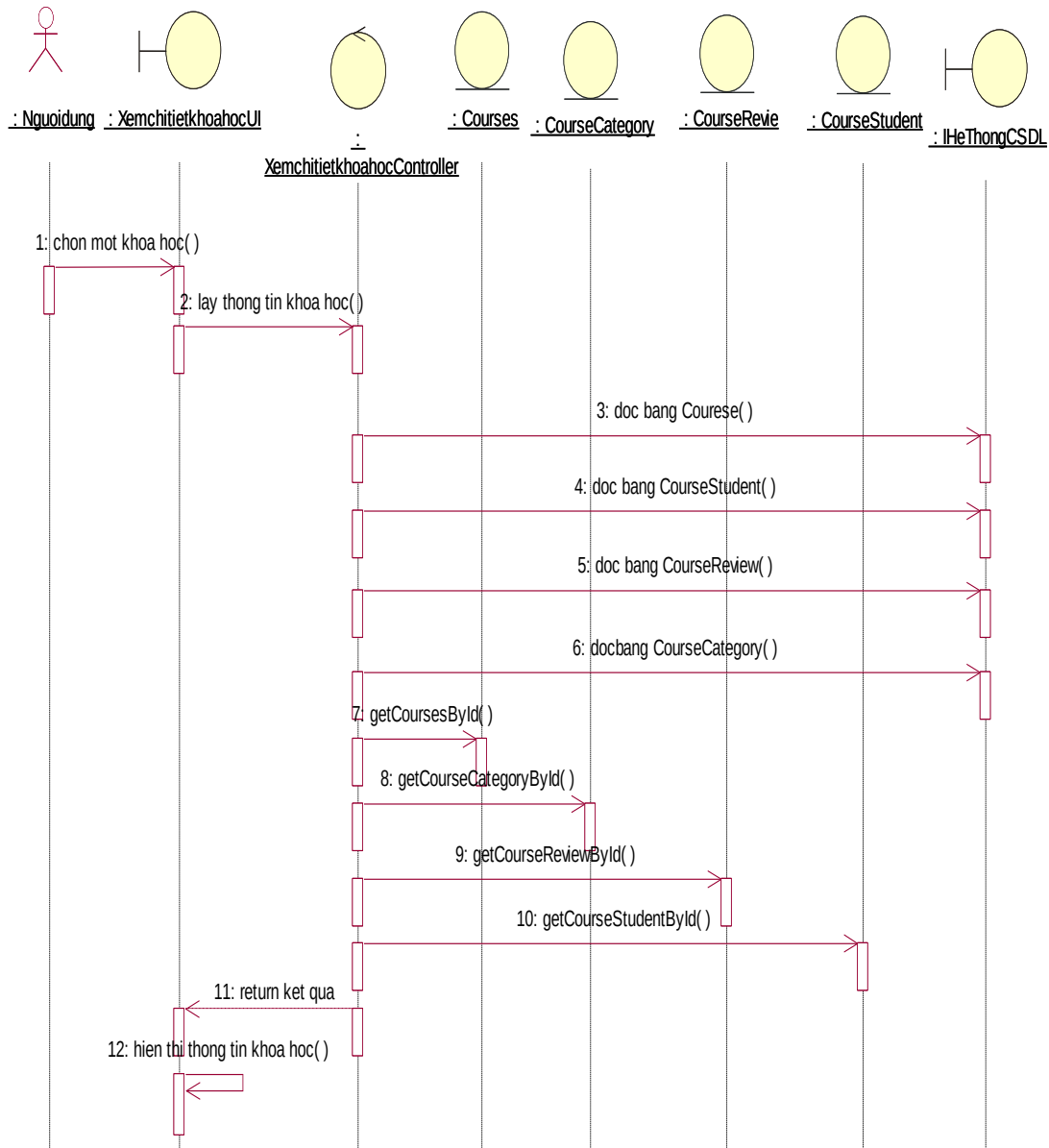
Hình 2.6. Biểu đồ trình tự use case xem chi tiết khoá học
