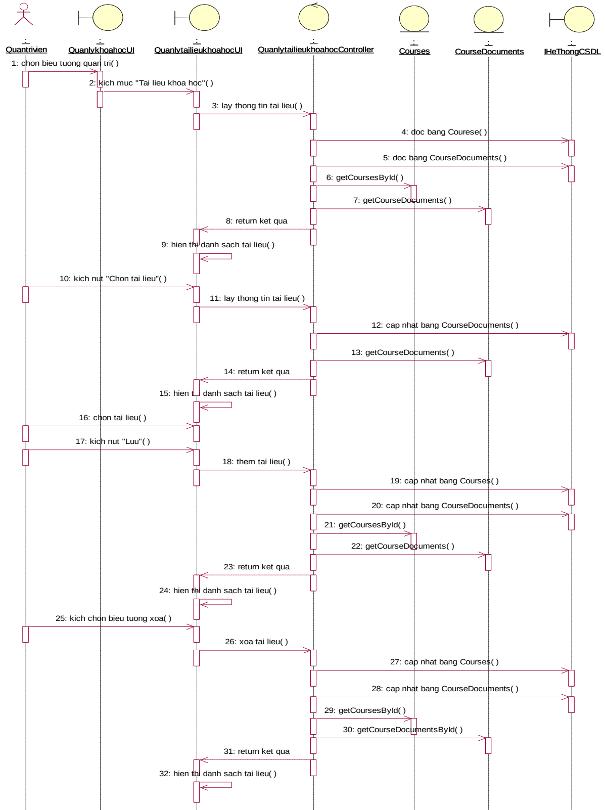
Hình 2.29. Biểu đồ trình tự use case quản lý tài liệu khóa học trong chi tiết khóa học
