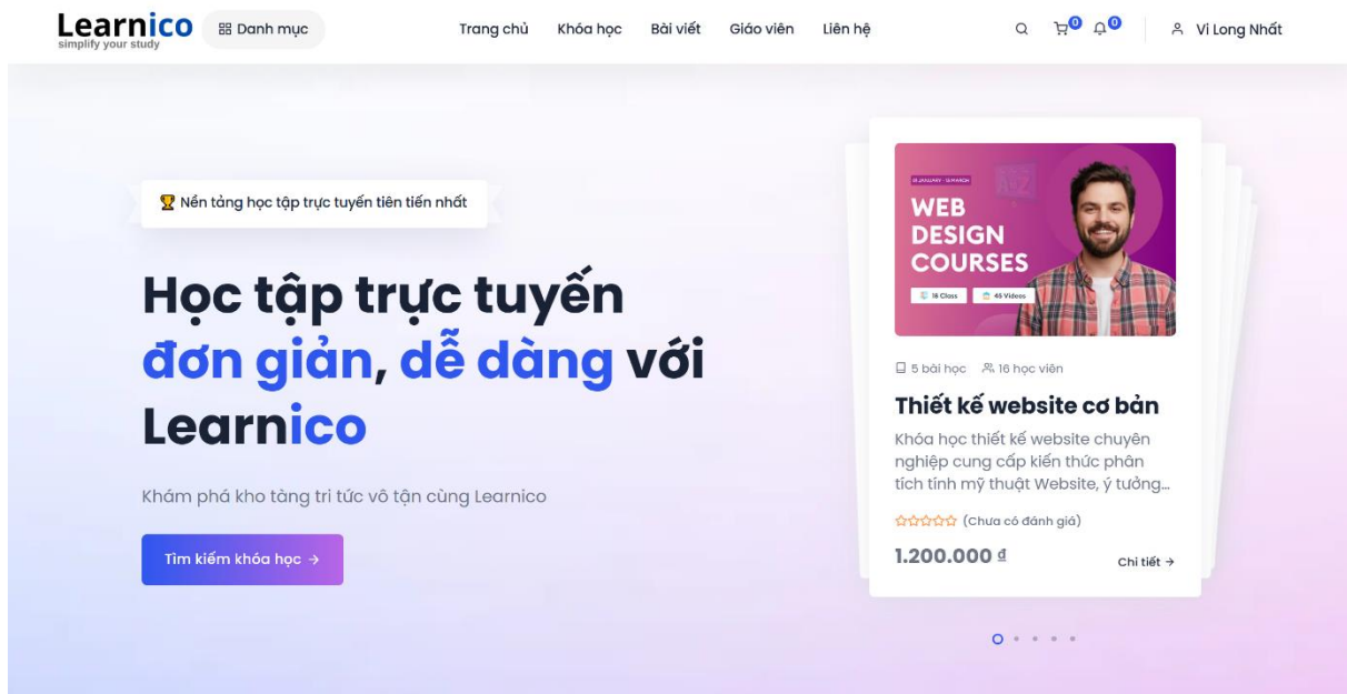
Hình 3.3. Giao diện trang chủ
