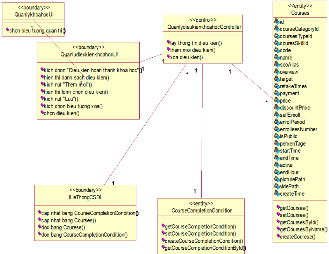
Hình 2.36. Biểu đồ lớp phân tích use case quản lý điều kiện hoàn thành khoá học trong chi tiết khoá học
