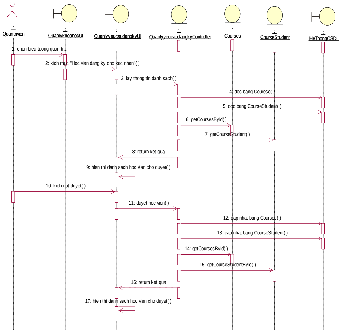
Hình 2.30. Biểu đồ trình tự use case quản lý yêu cầu đăng ký của học viên trong chi tiết khoá học
