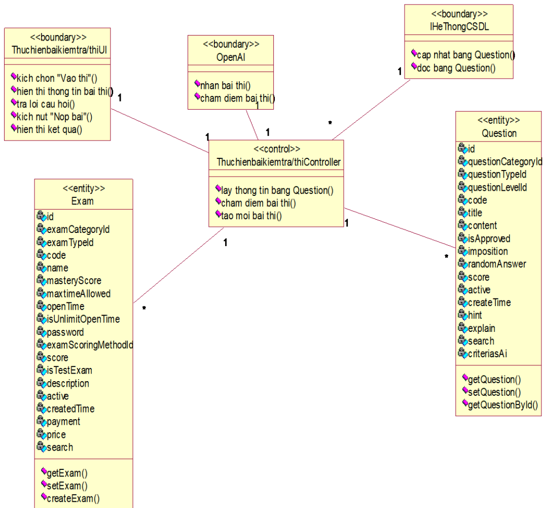
Hình 2.17. Biểu đồ lớp phân tích use case thực hiện bài kiểm tra/thi
