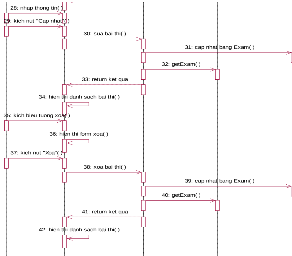
Hình 2.44. Biểu đồ trình tự use case quản lý bài kiểm tra/thi
