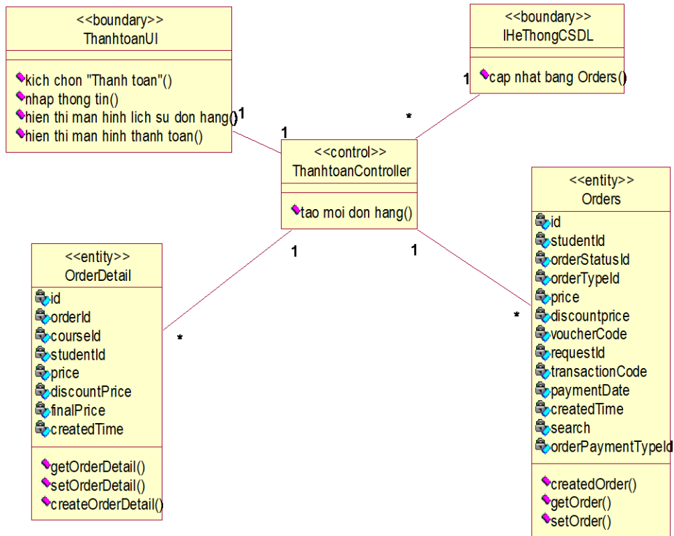
Hình 2.11. Biểu đồ lớp phân tích use case thanh toán
