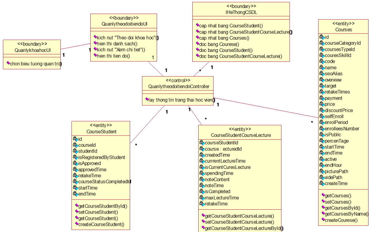
Hình 2.39. Biểu đồ lớp phân tích use theo dõi tiến độ của học viên trong chi tiết khoá học
