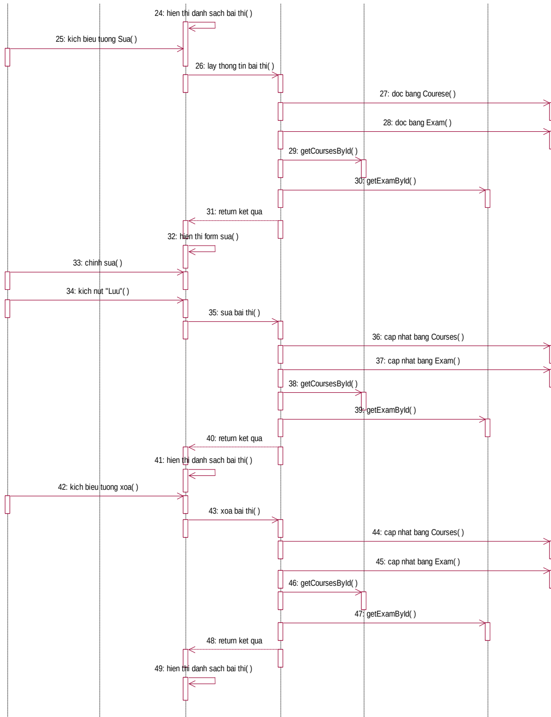
Hình 2.26. Biểu đồ trình tự use case quản lý bài kiểm tra/thi trong chi tiết khoá học
