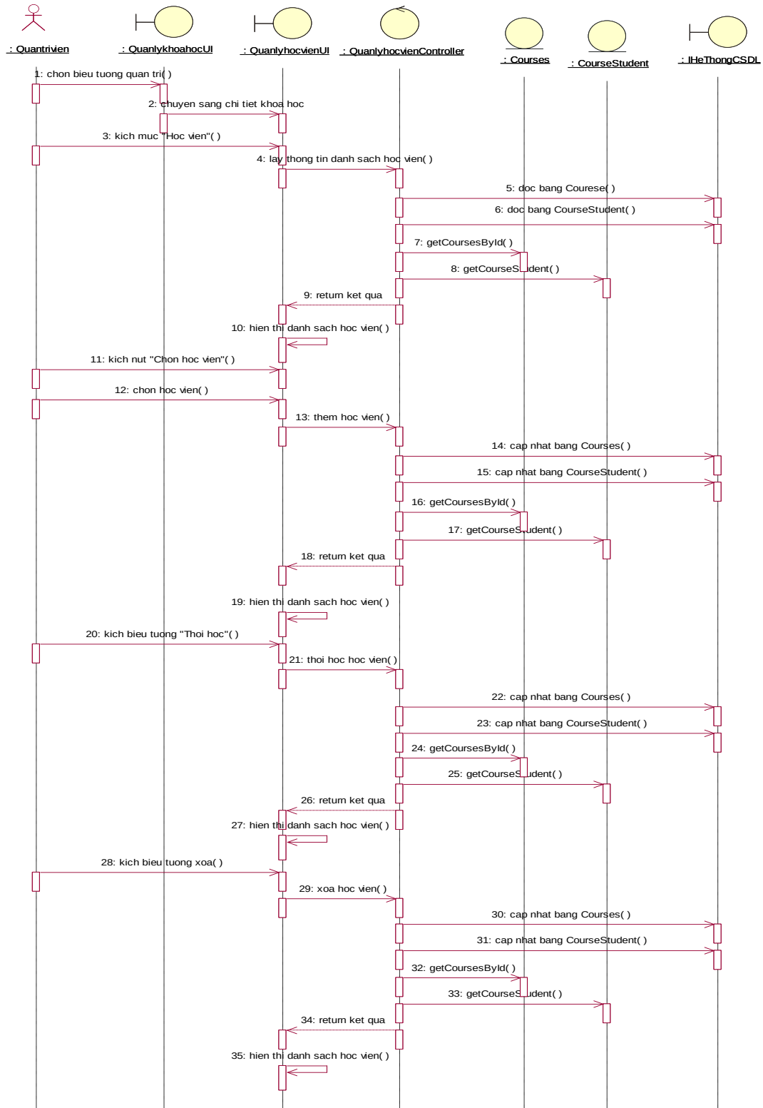
Hình 2.24. Biểu đồ trình tự use case quản lý học viên trong chi tiết khoá học
