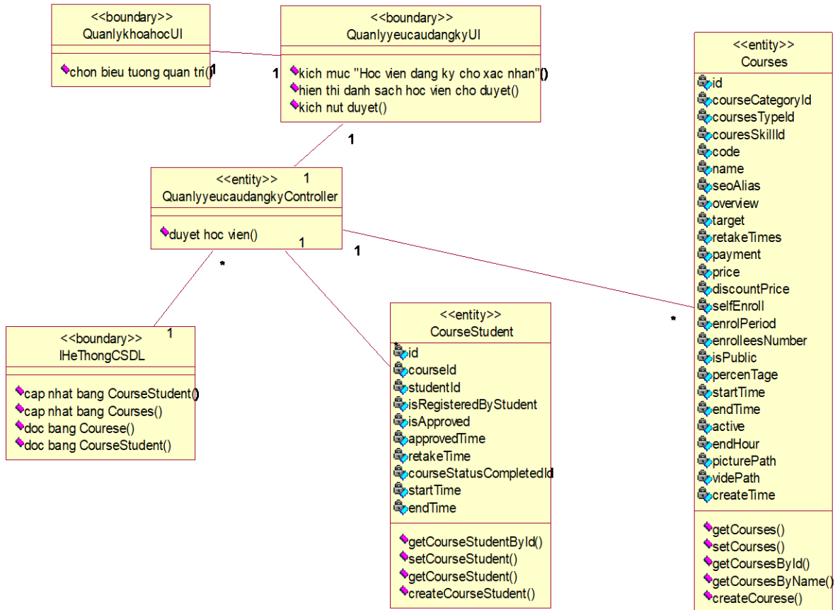
Hình 2.38. Biểu đồ lớp phân tích use case quản lý yêu cầu đăng ký của học viên trong chi tiết khoá học
