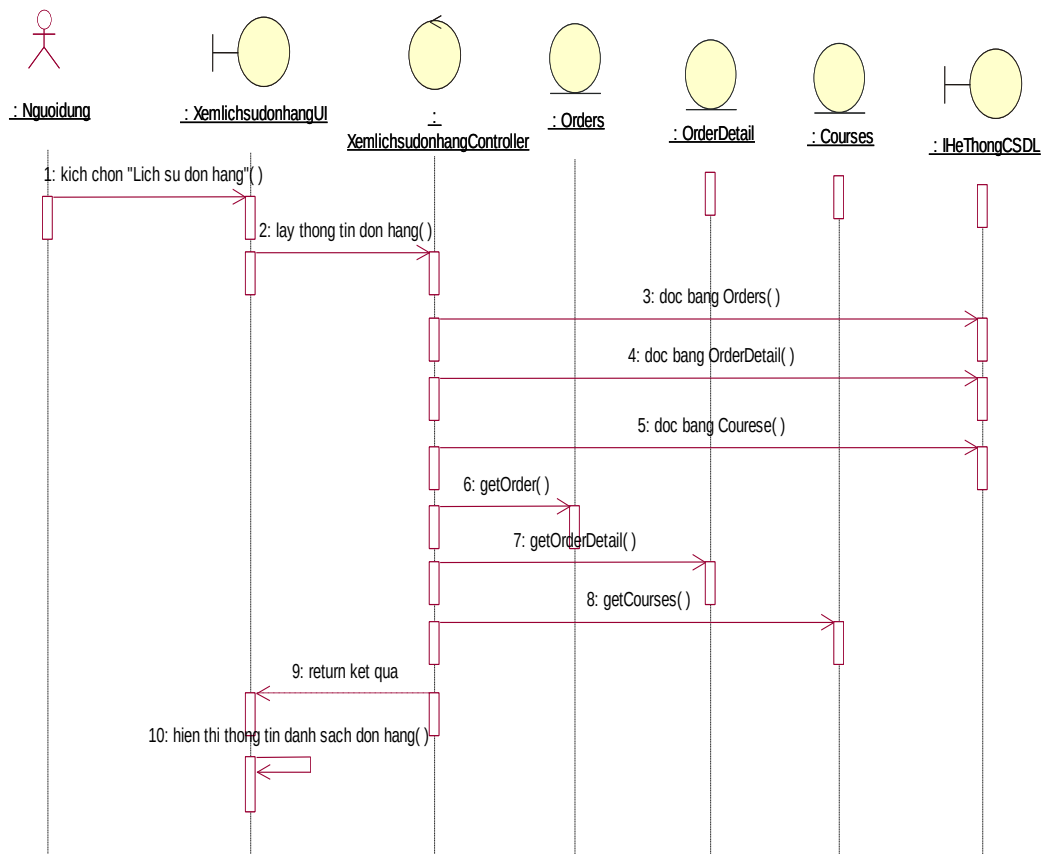
Hình 2.12. Biểu đồ trình tự use case xem lịch sử đơn hàng
