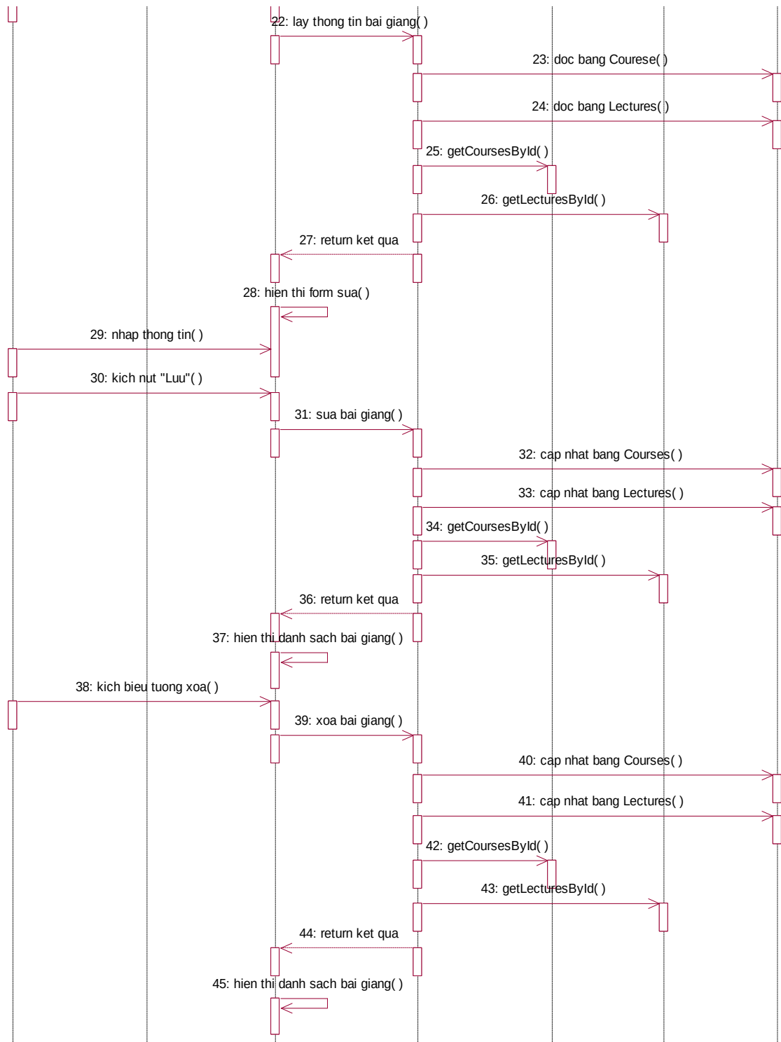
Hình 2.25. Biểu đồ trình tự use case quản lý bài giảng trong chi tiết khoá học
