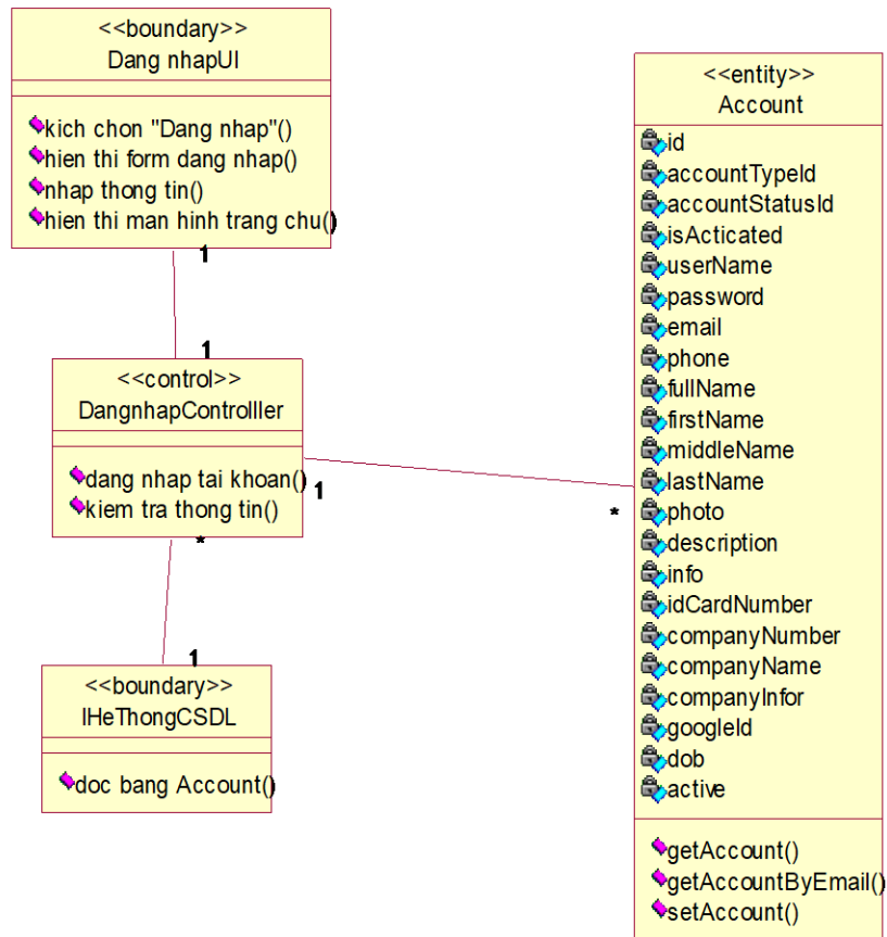
Hình 2.3. Biểu đồ lớp phân tích use case đăng nhập
