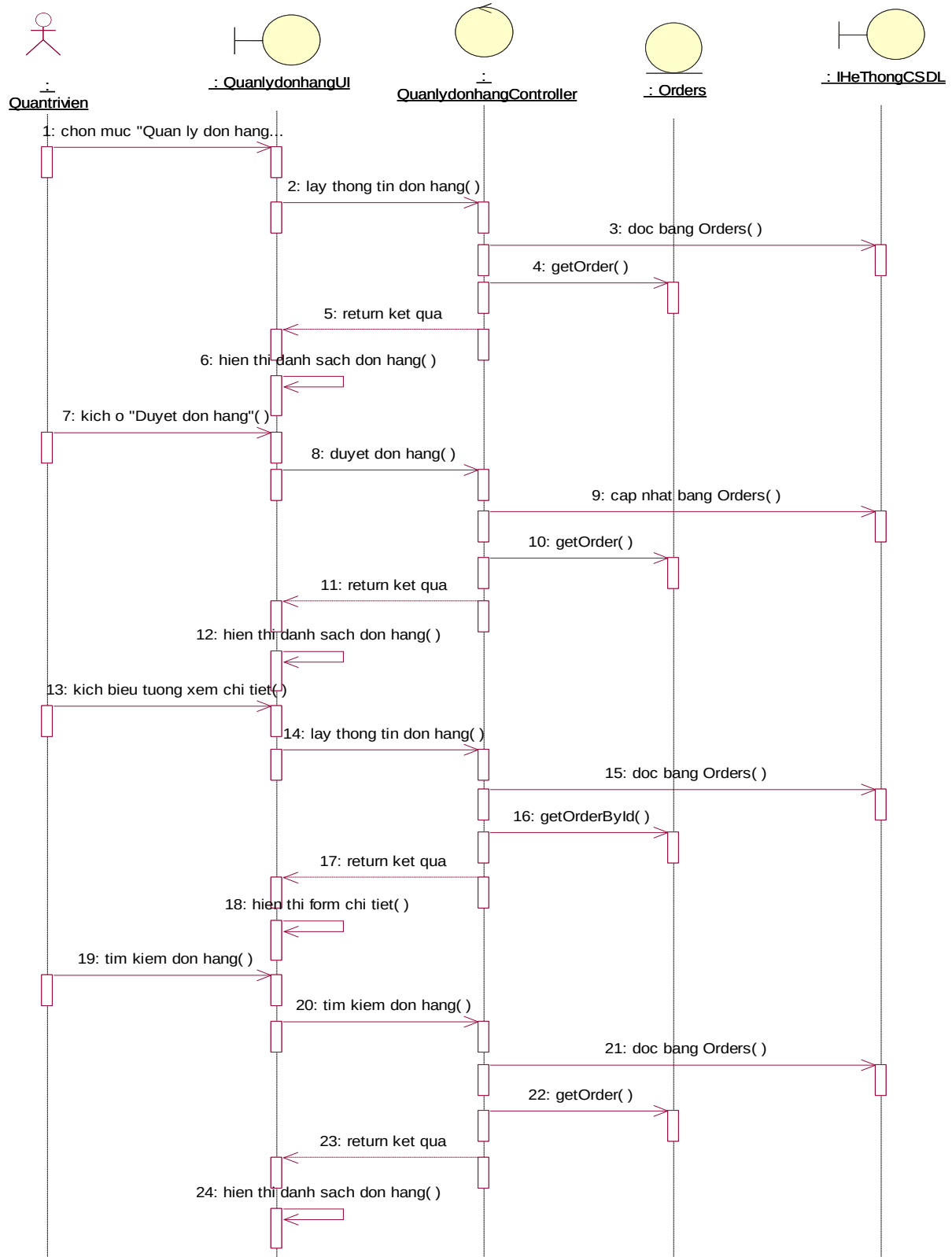
Hình 2.46. Biểu đồ trình tự use case quản lý đơn hàng
