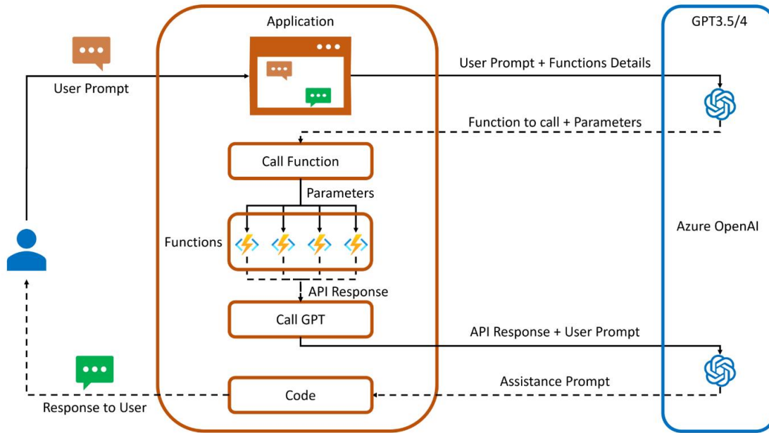
Hình 1.4. Sơ đồ hoạt động của OpenAI GPT
