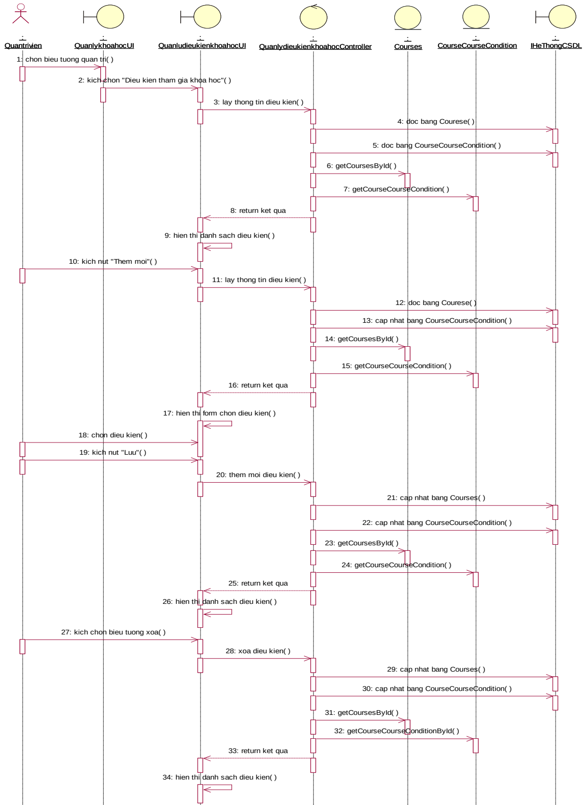
Hình 2.27. Biểu đồ trình tự use case quản lý điều kiện tham gia khóa học trong chi tiết khóa học
