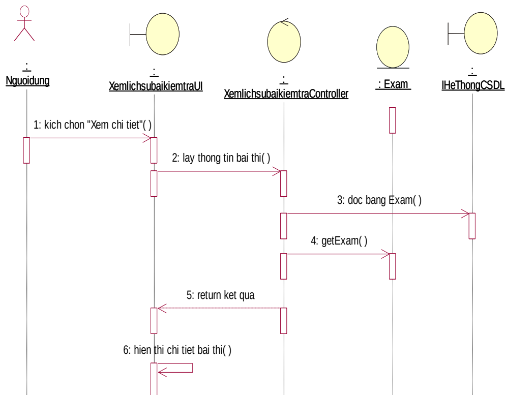
Hình 2.18. Biểu đồ trình tự use case xem lịch sử bài kiểm tra/thi
