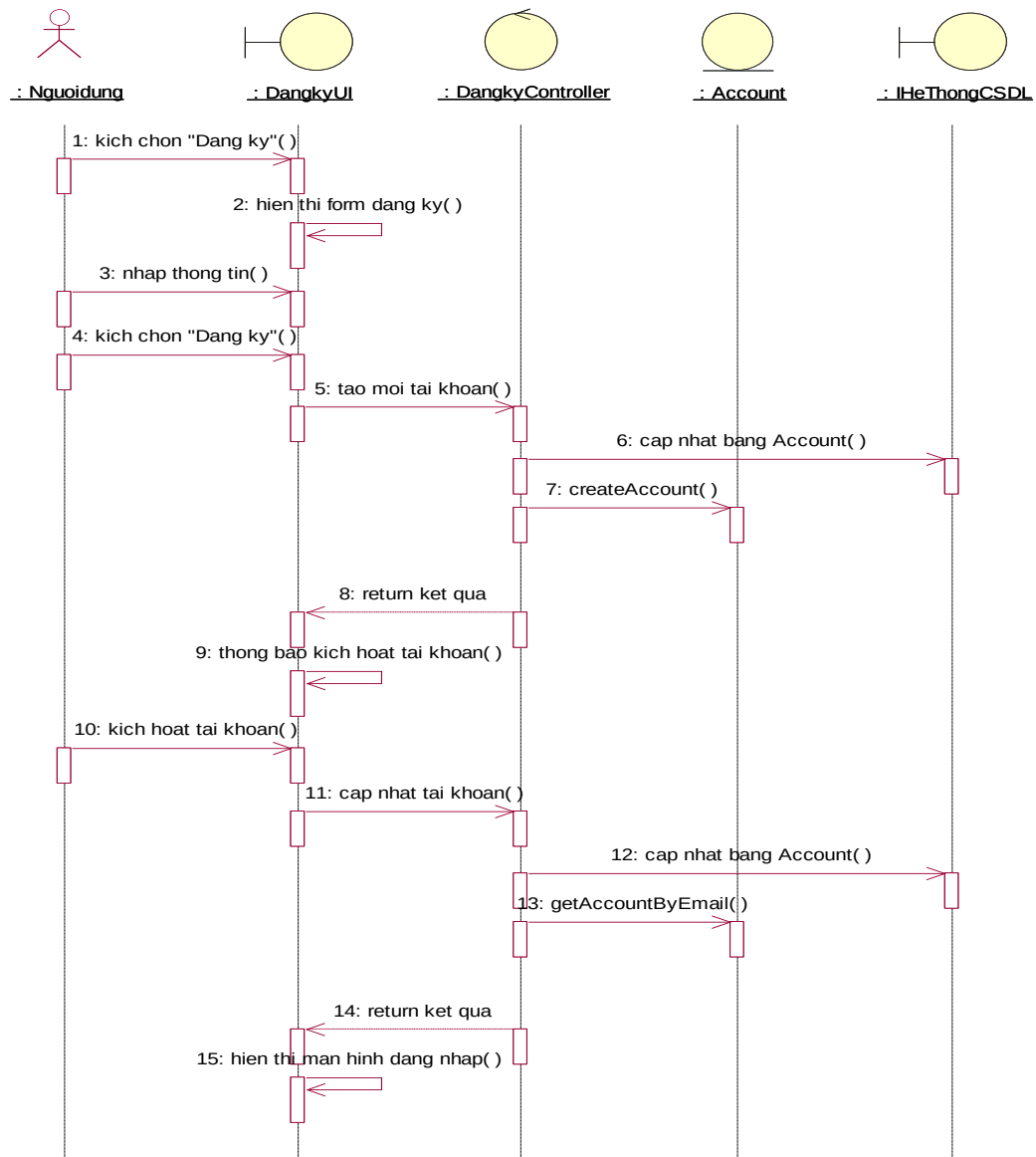
Hình 2.4. Biểu đồ trình tự use case đăng ký
