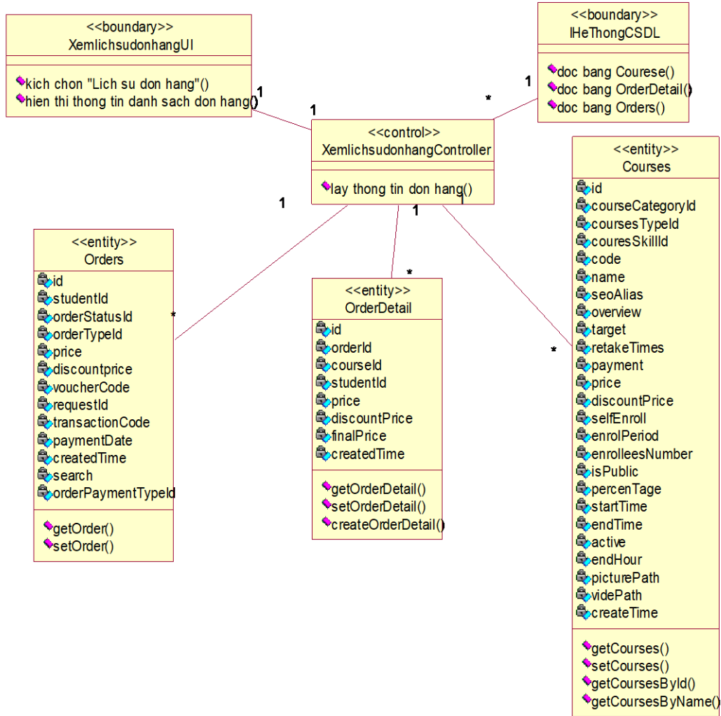
Hình 2.13. Biểu đồ lớp phân tích use case xem lịch sử đơn hàng
